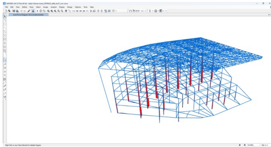
Sforzo normale – combinazione di carico SLU_fondamentale
