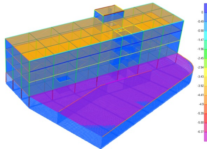
Figura 25-distribuzione dei carichi permanenti strutturali G1_blocco3
