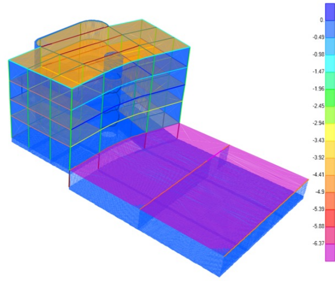
Figura 18-distribuzione dei carichi permanenti strutturali G1_blocco 2
