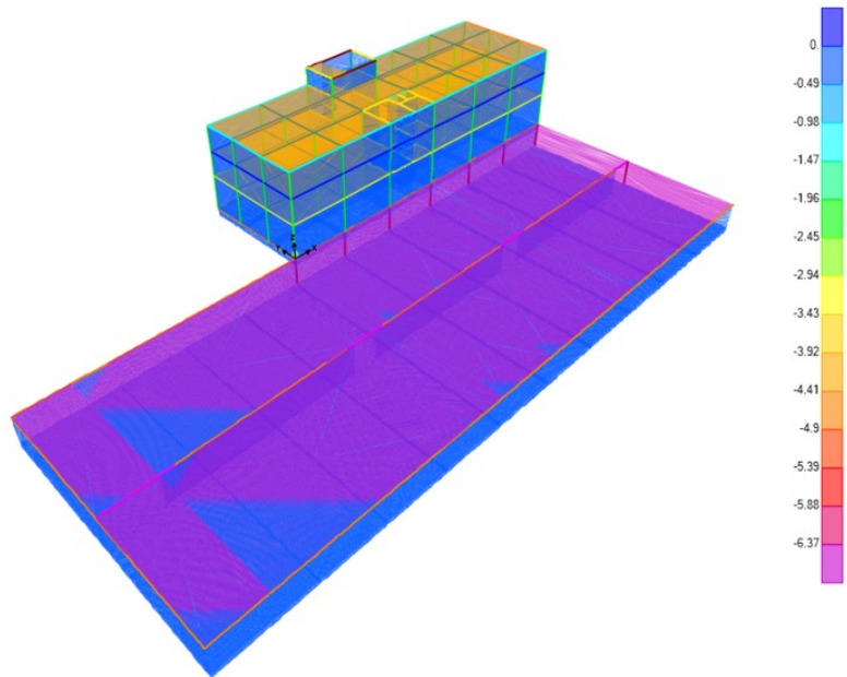
Figura 12-distribuzione dei carichi permanenti strutturali G1_blocco1
