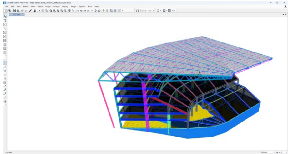
Modello - vista estrusa
