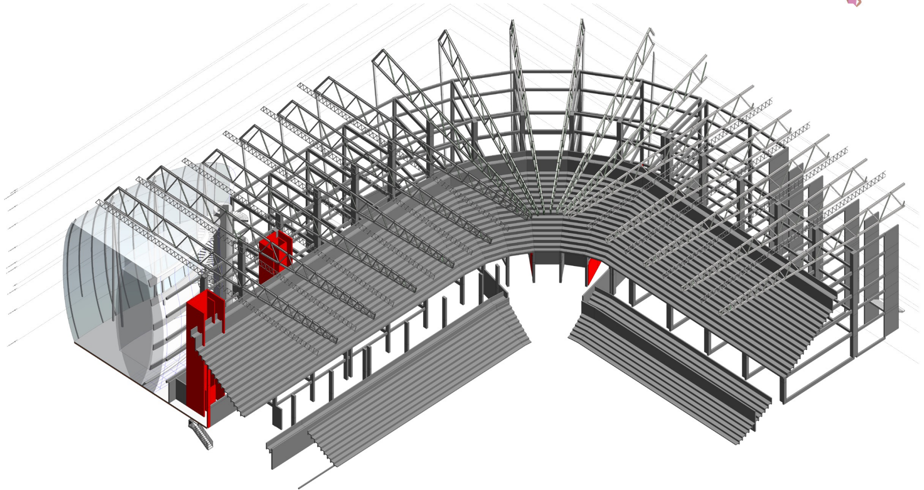
VISTA STRUTTURALE INTERNA DAL CAMPO TRIBUNA OVEST LATERALE
