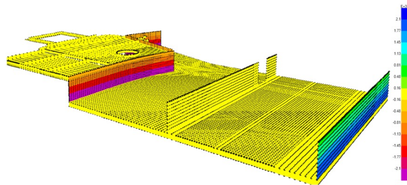
Figura 24-spinta del terreno QT_blocco 2
