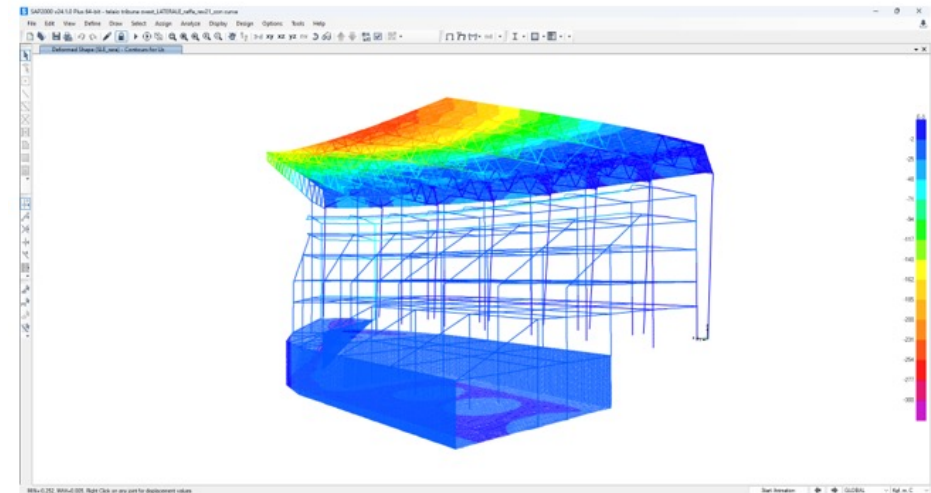
Deformata - combinazione SLE_rara
