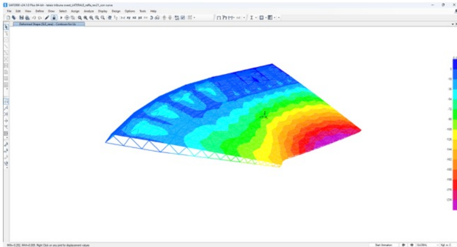
Deformata solo copertura - combinazione SLE_rara
