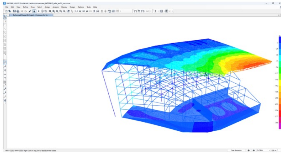
Deformata - combinazione SLE_rara
