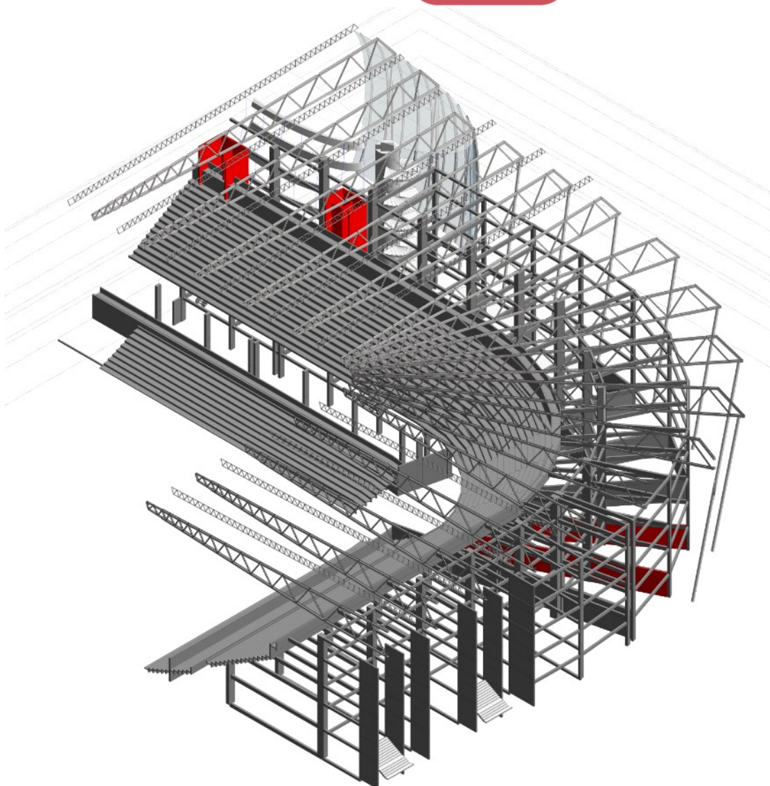
VISTA STRUTTURALE ESTERNA TRIBUNA OVEST LATERALE
