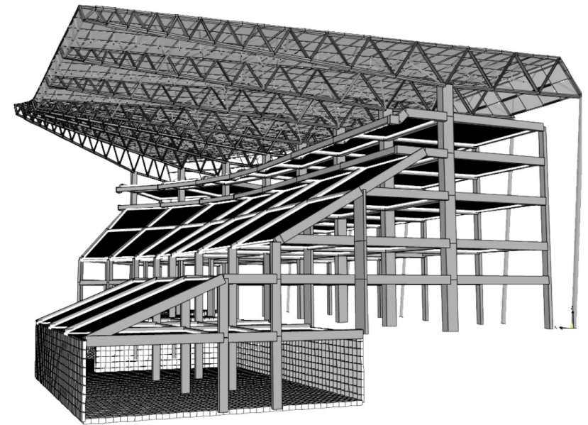
SEZIONE TRIBUNA OVEST CENTRALE
